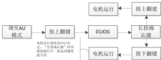
图 6-5 点动运行流程图
