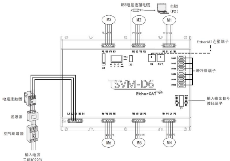
图 2-1 TSVM-D6 系列交流伺服驱动器配线图
