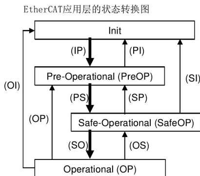
图 8-1 状态转换图
