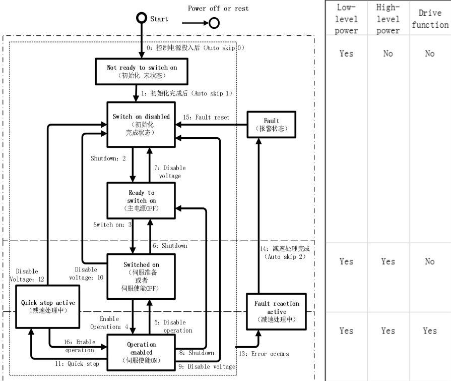
图 8-2 状态转换图
