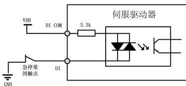
图 3-2 外接急停示意图
