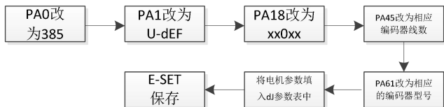
图 6-2 设置电机参数流程图
