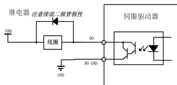
图 3-3 外接输出点示意图
