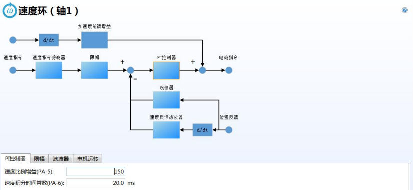
图 5-8 速度环参数表
