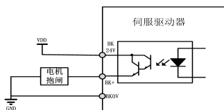
图 3-1 抱闸连接示意图
