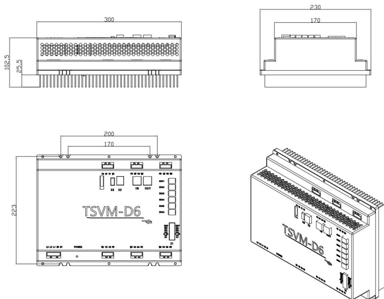
图 2-4 TSVM-D6- (10B、20) 产品外形与安装尺寸 (单位 mm)
