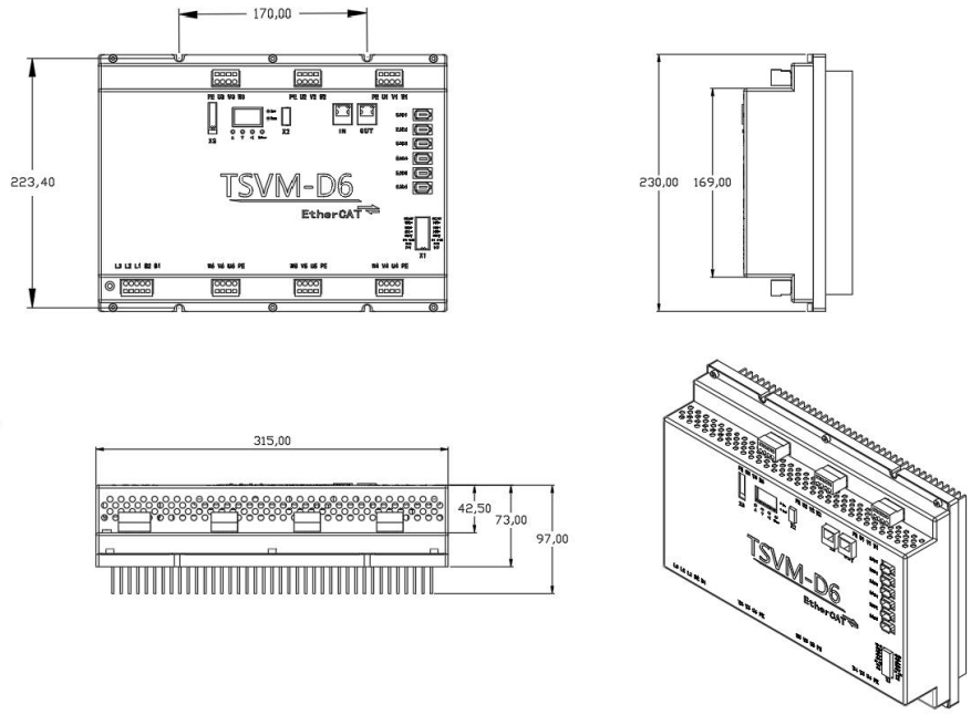
图 2-3 TSVM-D6- (6A、6B) 产品外形与安装尺寸 (单位 mm)
