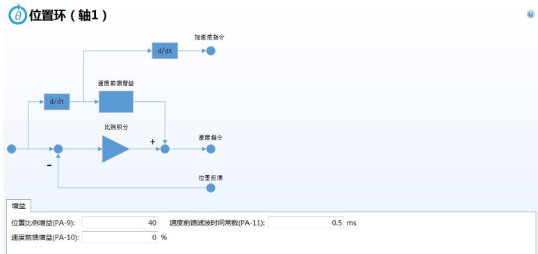
图 11- 21 位置环参数表
