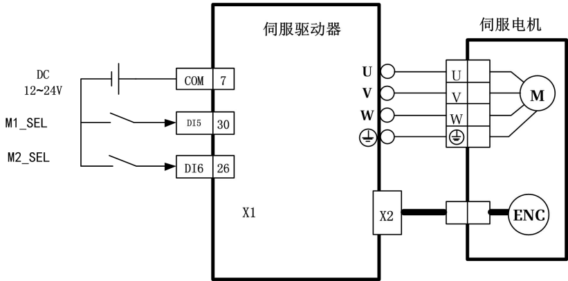
图 7-6 模式切换接线示意图
