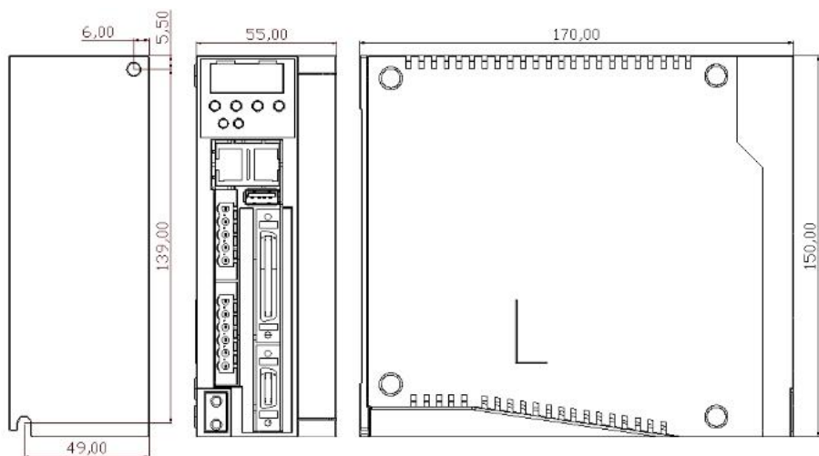
图 3-3 TSVB-□□015L 产品外形与安装尺寸 (单位 mm)
