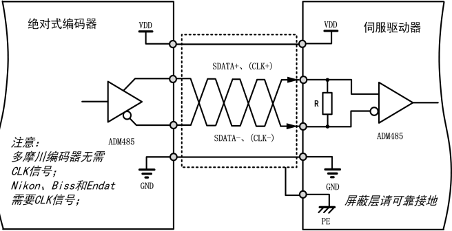
图 3-16 绝对式编码器输入信号接口电路
