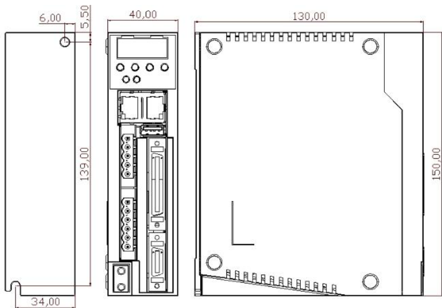
图 3-1 TSVB-□□005L 产品外形与安装尺寸（单位 mm）
