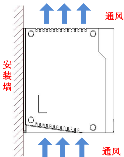
图 3-6 TSVB 系列交流伺服驱动器安装方向
