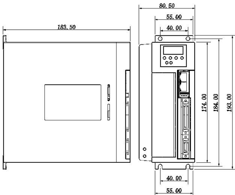
图 3-4 TSVB-□□020L/TSVB-□□030L 产品外形与安装尺寸 (单位 mm)
