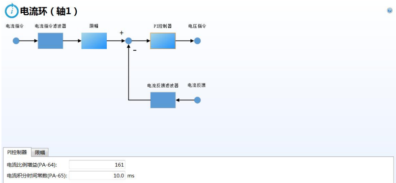
图 11- 18 电流环参数表
