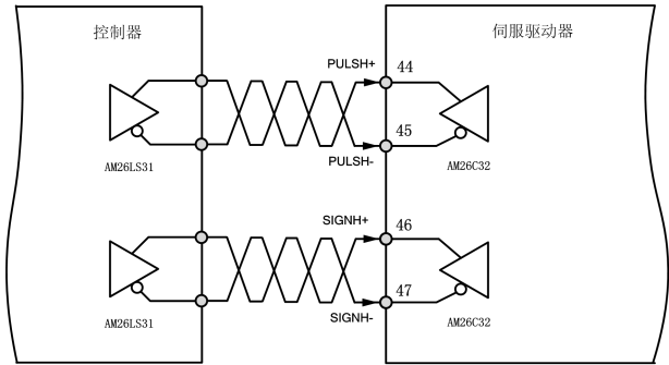
图 3-12 高速脉冲差分输入脉冲和方向接口电路
