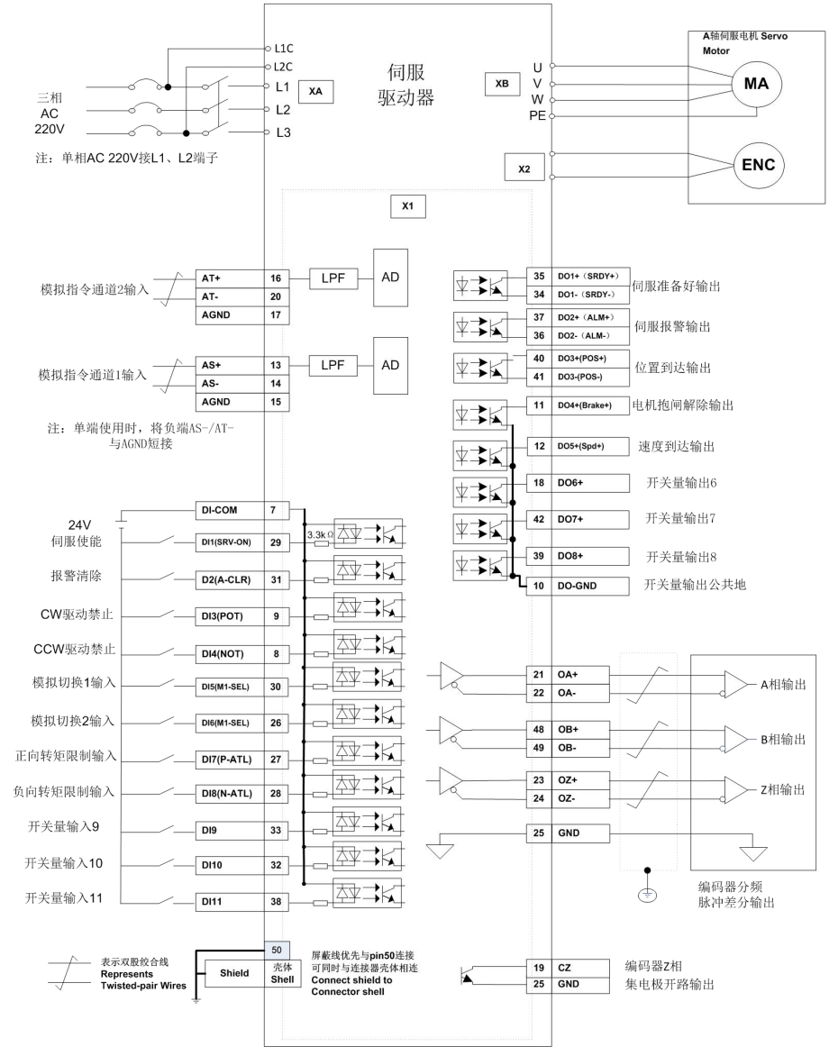
图 3-20 模拟速度/转矩指令控制方式接线图
