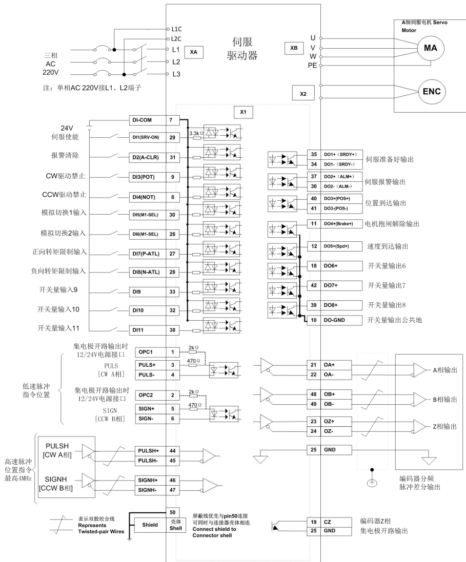
图 3-19 位置控制方式接线图
