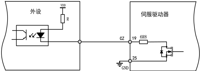
图 3-13 编码器 Z 信号集电极开路输出
