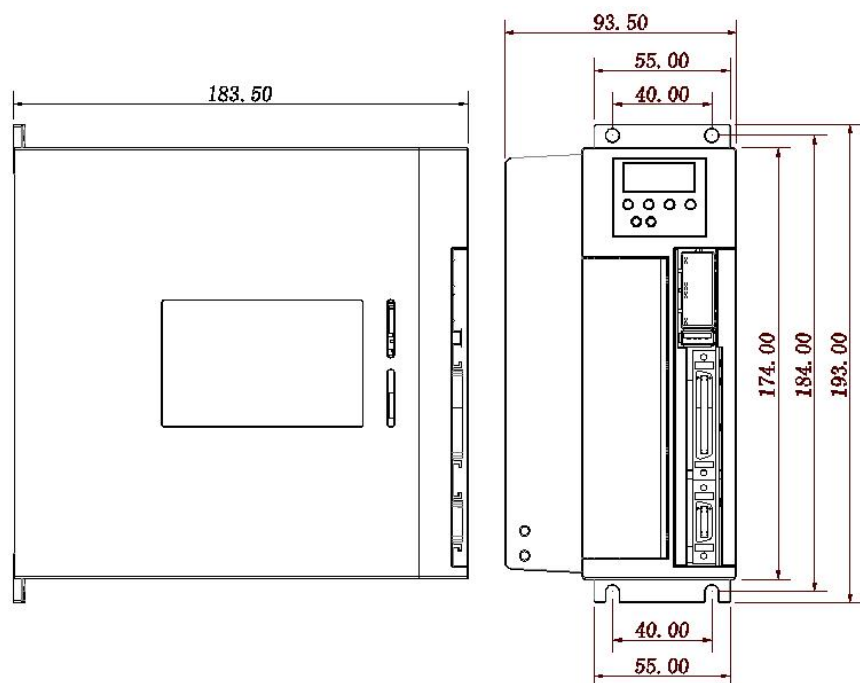
图 3-5 TSVB-□□050L 产品外形与安装尺寸 (单位 mm)
