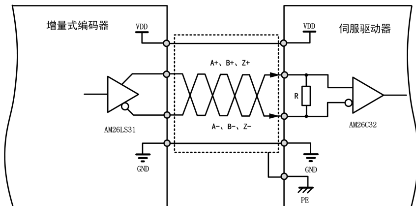
图 3-15 省线式编码器输入信号接口电路
