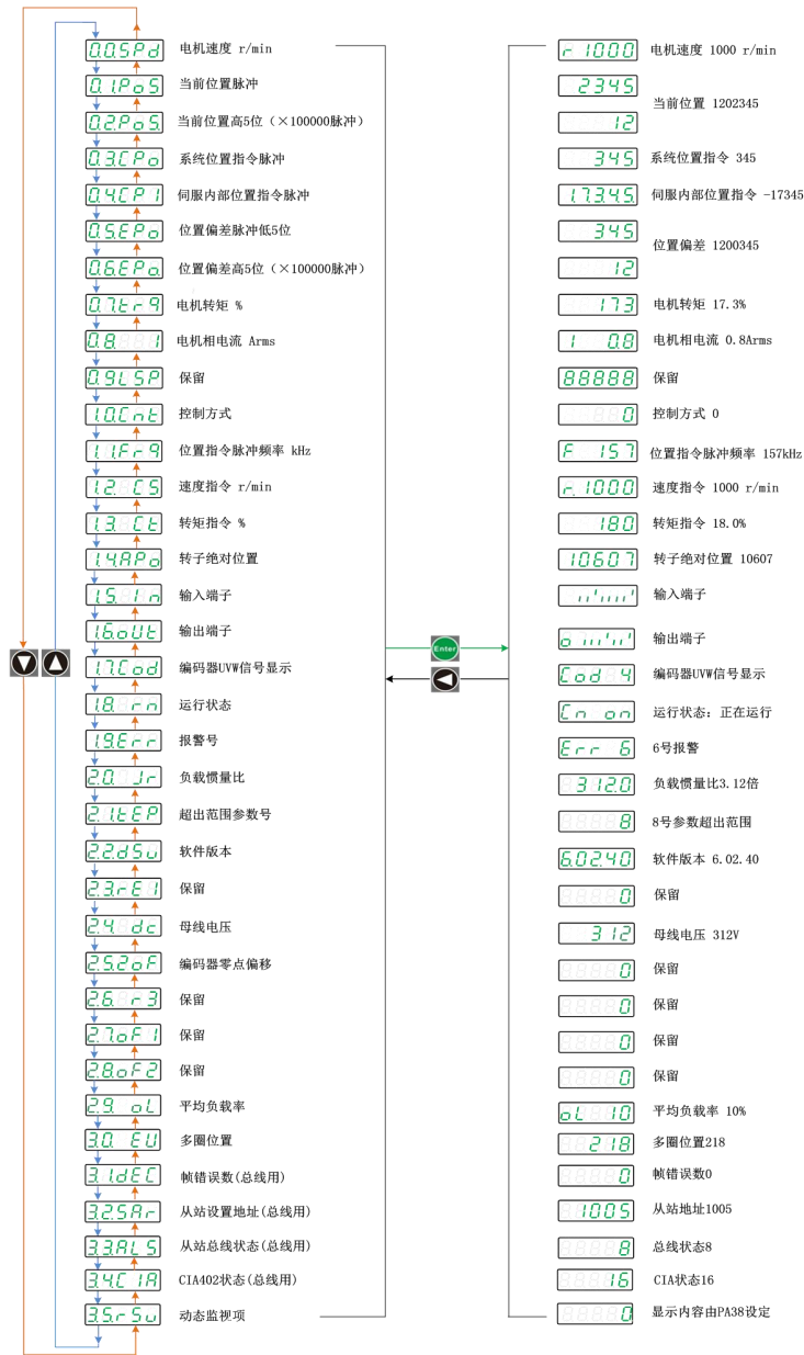
图 4-3 二级菜单
