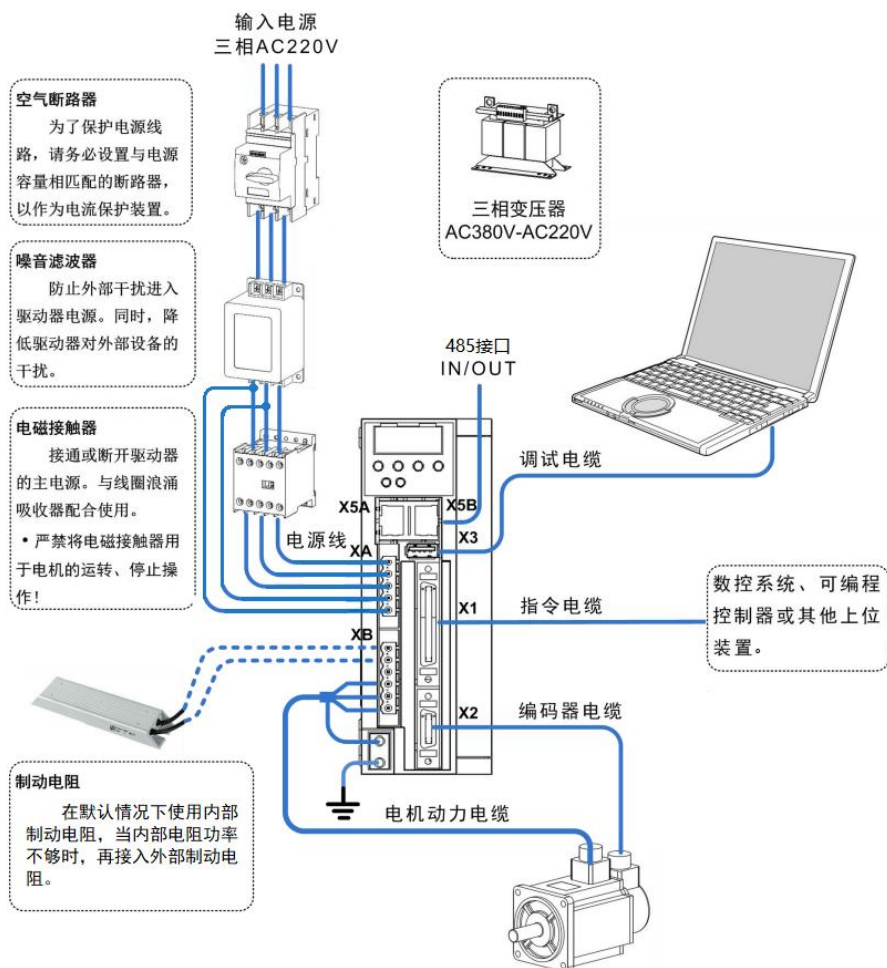
图 3-8 TSVB 脉冲系列交流伺服驱动器配线图
