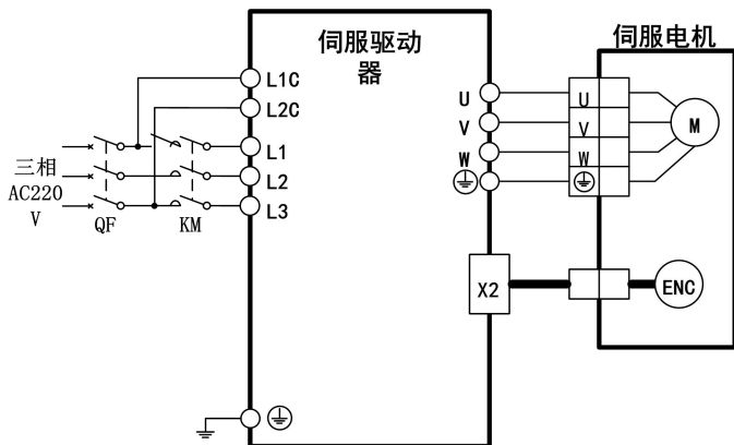
图 5- 1 驱动器接线图
