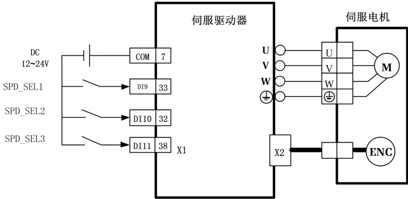
图 7-7 多段速度控制接线示意图
