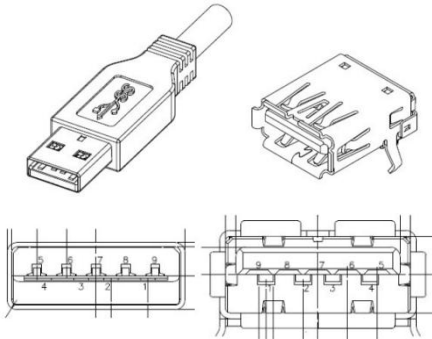
图 3- 17 USB3.0 A 型 USB 插头（左）和插座（右）
