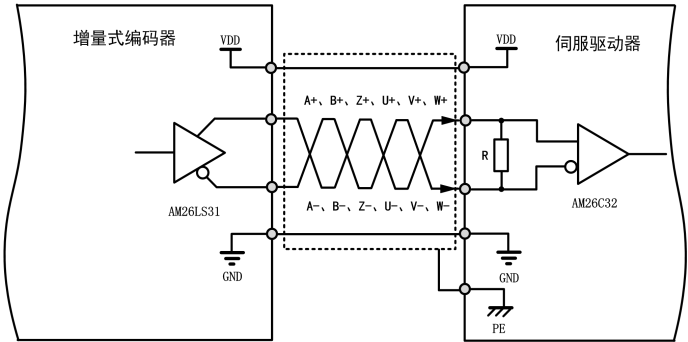
图 3-14 增量式编码器输入信号接口电路
