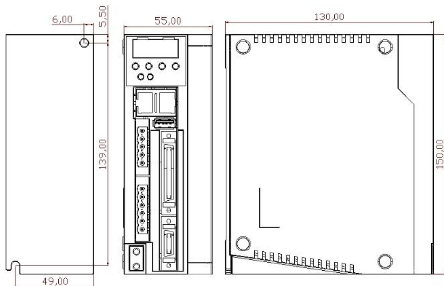
图 3-2 TSVB-□□010L 产品外形与安装尺寸（单位 mm）
