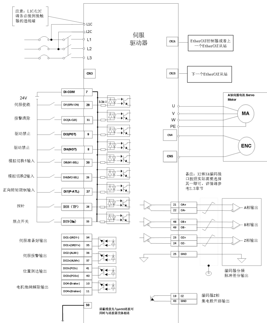
图 3-10 TSVC-EA 系列控制接线连接图
