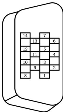
图 3-8 CN3 焊线端脚号图
