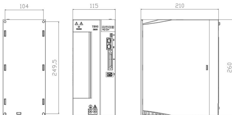
图 2-6 TSVC-EA050H/75H 产品外形与安装尺寸 (单位 mm)
