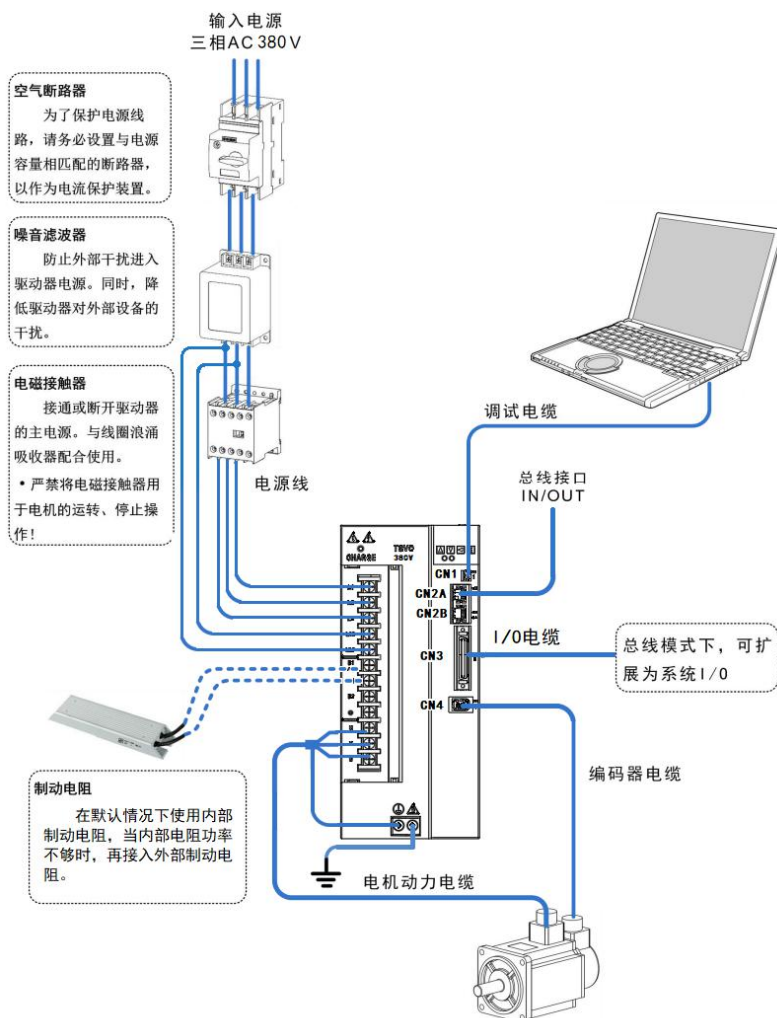
图 2-1 TSVC-EA-H (380V) 系列交流伺服驱动器配线图
