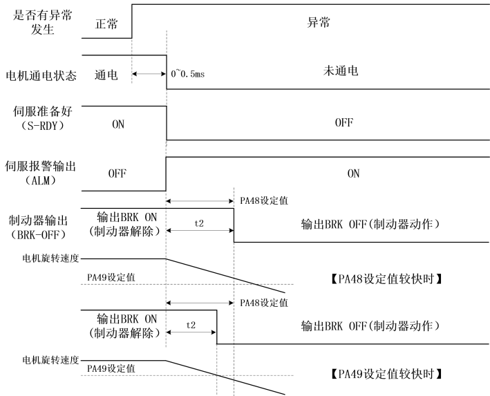
图 5-6 报警时序
