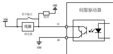
图 3-7 抱闸接线示意图
