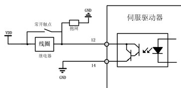
图 3-7 抱闸接线示意图
