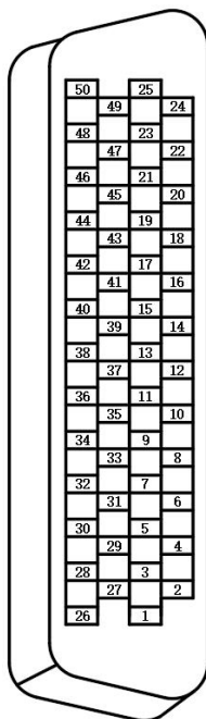
图 3-6 CN3 焊线端脚号图
