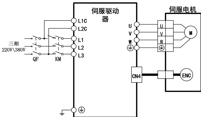
图 5-1 驱动器接线图
