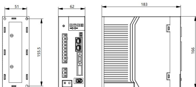
图 2-4 TSVC-EA030L (220V) / 015H (380V) 产品外形与安装尺寸 (单位 mm)
