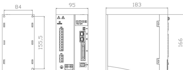
图 2-5 TSVC-EA025H/035H 产品外形与安装尺寸 (单位 mm)
