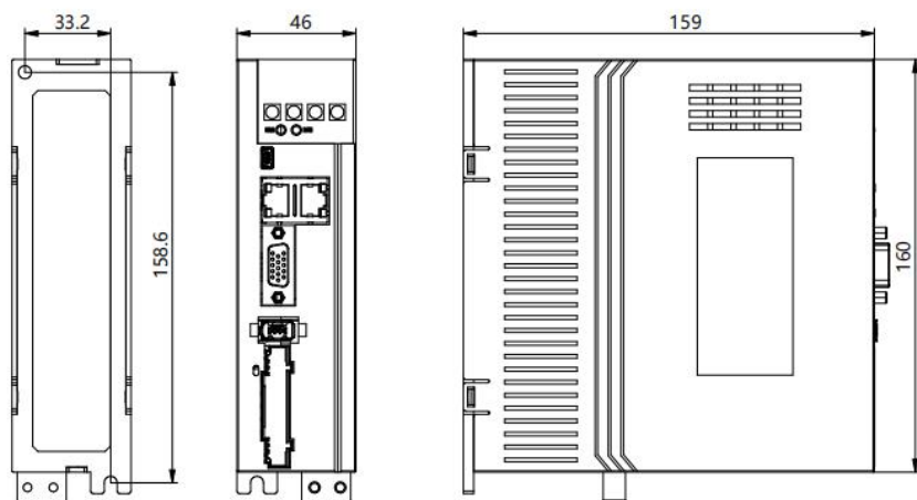
图 2-3 TSVC-EA010L、TSVC-EA015L 产品外形与安装尺寸（单位 mm）
