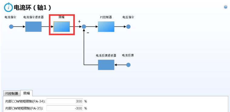
图 12-17 切换至限幅标签页的电流环界面
