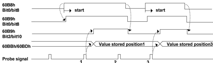
Negative edge 的情况
