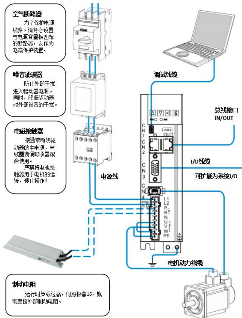
图 2-1 TSVC-EA 系列交流伺服驱动器配线图
