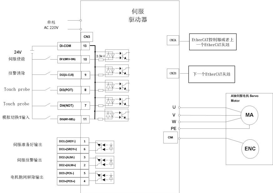
图 3-5 TSVC-EA 系列控制接线连接图
