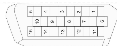
图 3-2 CN3 焊线端脚号图
