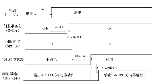
图 5-4 电源接通时接收伺服开启信号的时序
