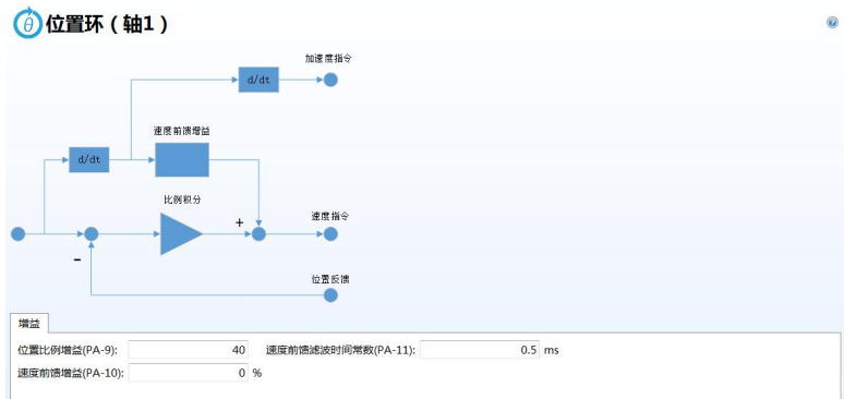
图 12- 19 位置环参数表
