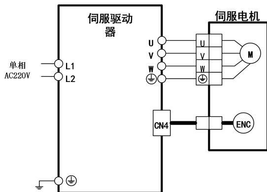
图 5-1 驱动器接线图
