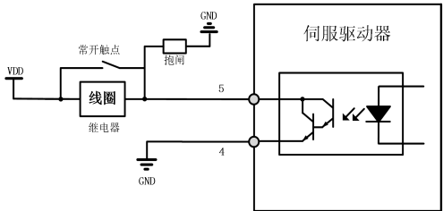
图 3-3 抱闸接线示意图
