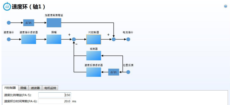
图 12- 18 速度环参数表
