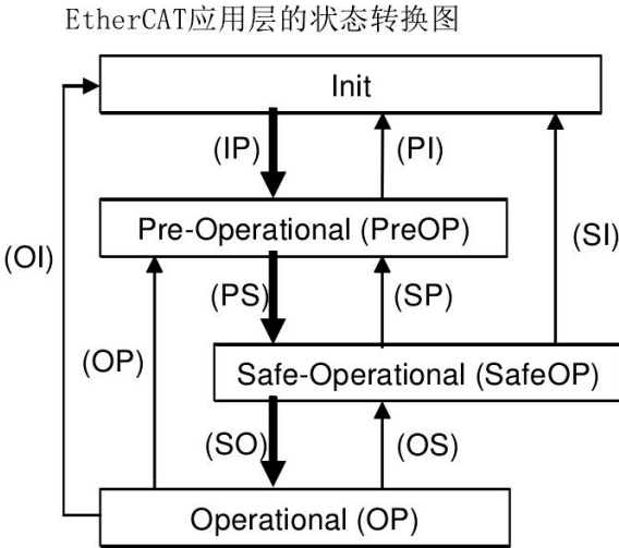
图 6-3 状态转换图
