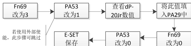
图 7-3 惯量识别流程图
