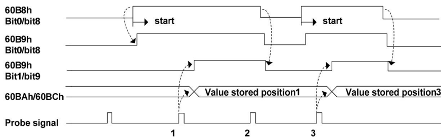
Positive edge 的情况
