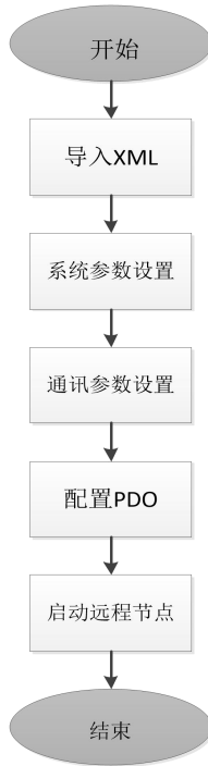
图 6-2 EtherCAT 使用设置流程图
