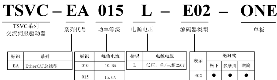
图 2-2 TSVC-EA 系列交流伺服驱动器命名规则
