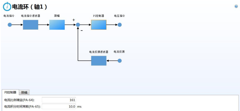
图 12- 16 电流环参数表
