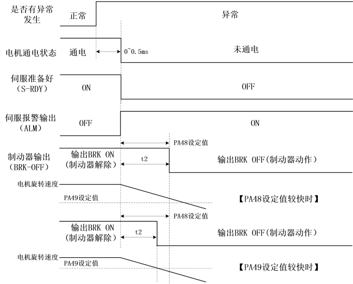
图 5-6 报警时序
