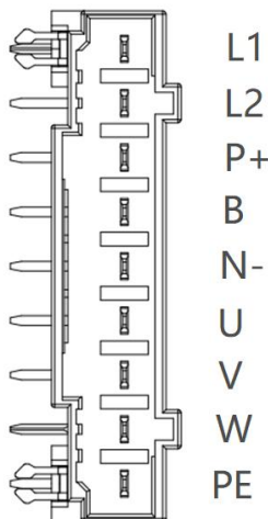
图 3-1 端子排分布图
