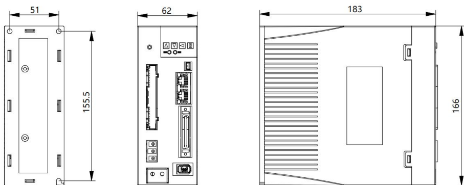
图 2-3 TSVC-PA030L (220V) / 015H (380V) 产品外形与安装尺寸 (单位 mm)
