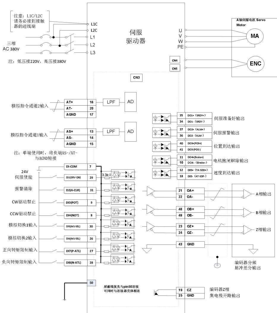
图 3-12 模拟速度/转矩指令控制方式接线图
