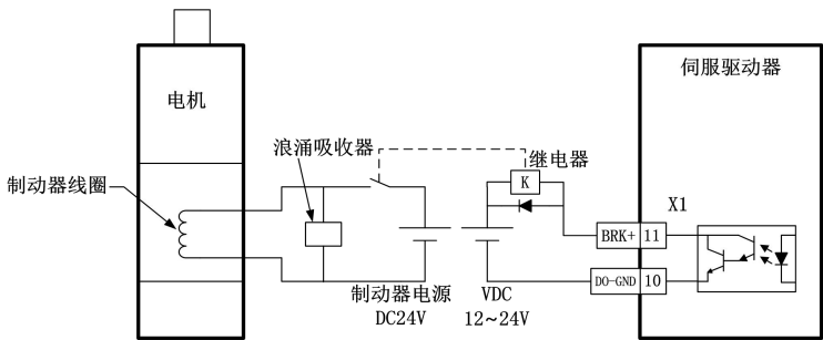
图 5-9 电磁制动器接线图
