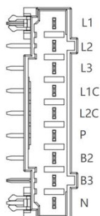
图 3-1 端子排分布图
