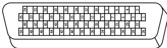
图 3-6 CN3 焊线端脚号图
