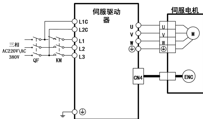
图 5-1 驱动器接线图
