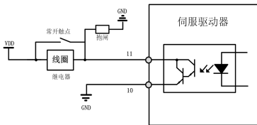
图 3-8 抱闸接线示意图
