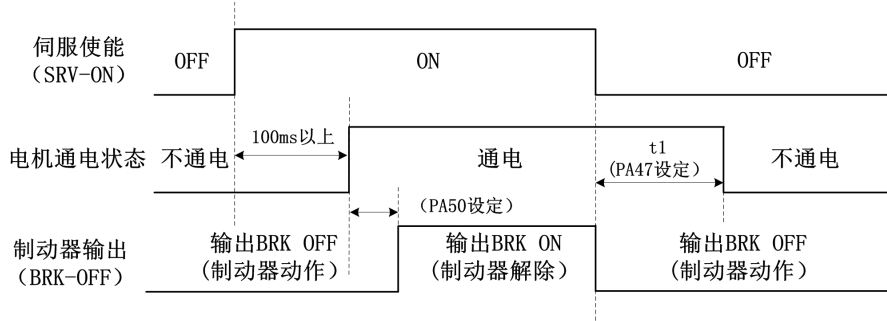
图 5-10 电源接通时接收伺服开启信号的时序
