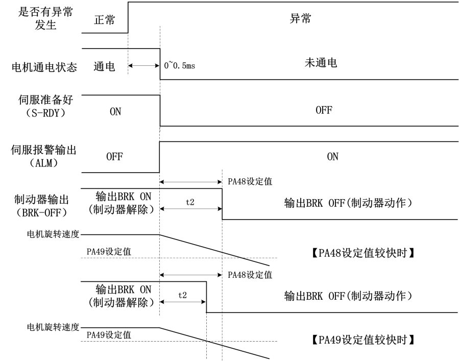
图 5-12 报警时序
