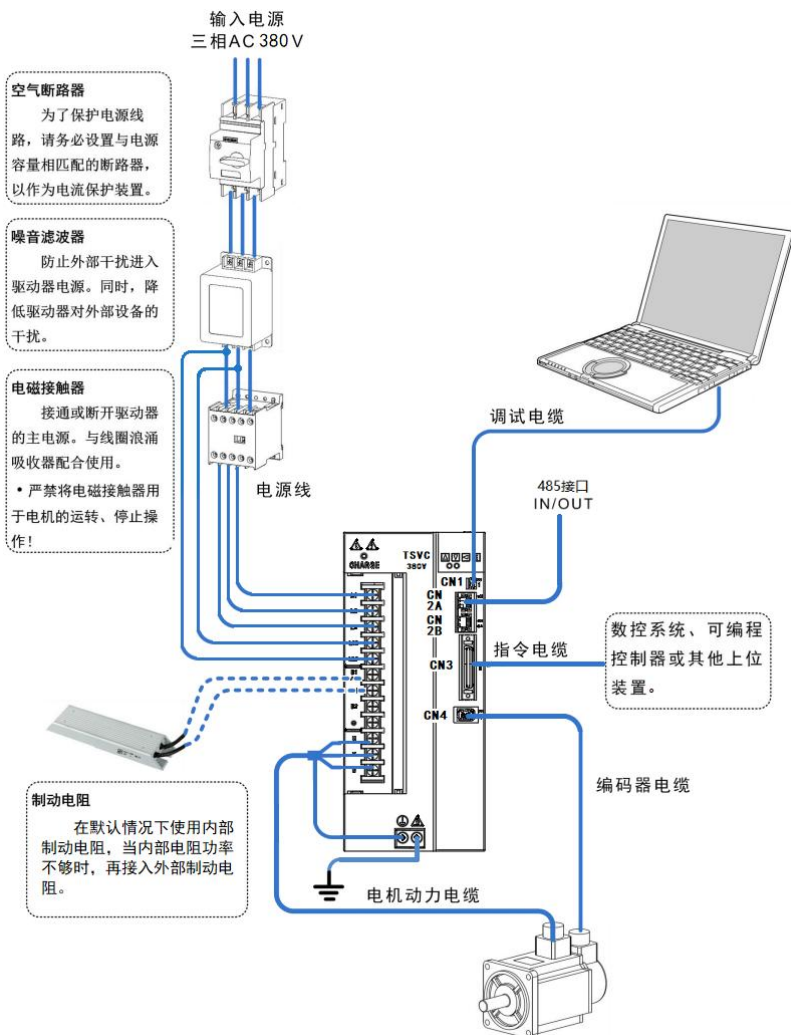
图 2-1 TSVC-PA-H（380V）脉冲系列交流伺服驱动器配线图
