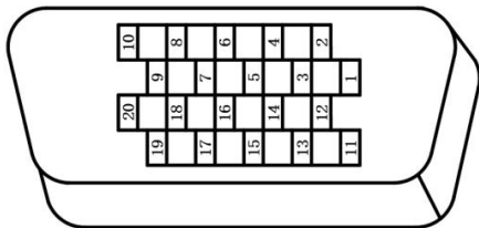
图 3-10 CN5 焊线端脚号图
