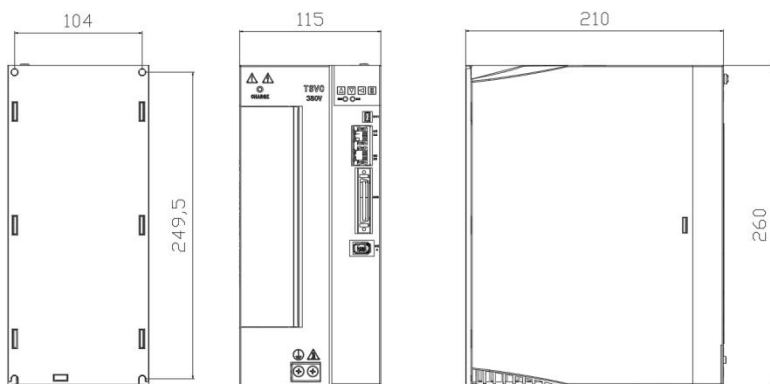
图 2-5 TSVC-PA050H/75H 产品外形与安装尺寸 (单位 mm)
