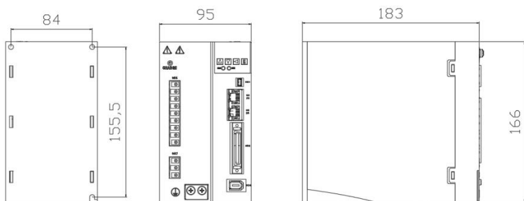
图 2-3 TSVC-PA030L (220V) / 015H (380V) 产品外形与安装尺寸 (单位 mm)
