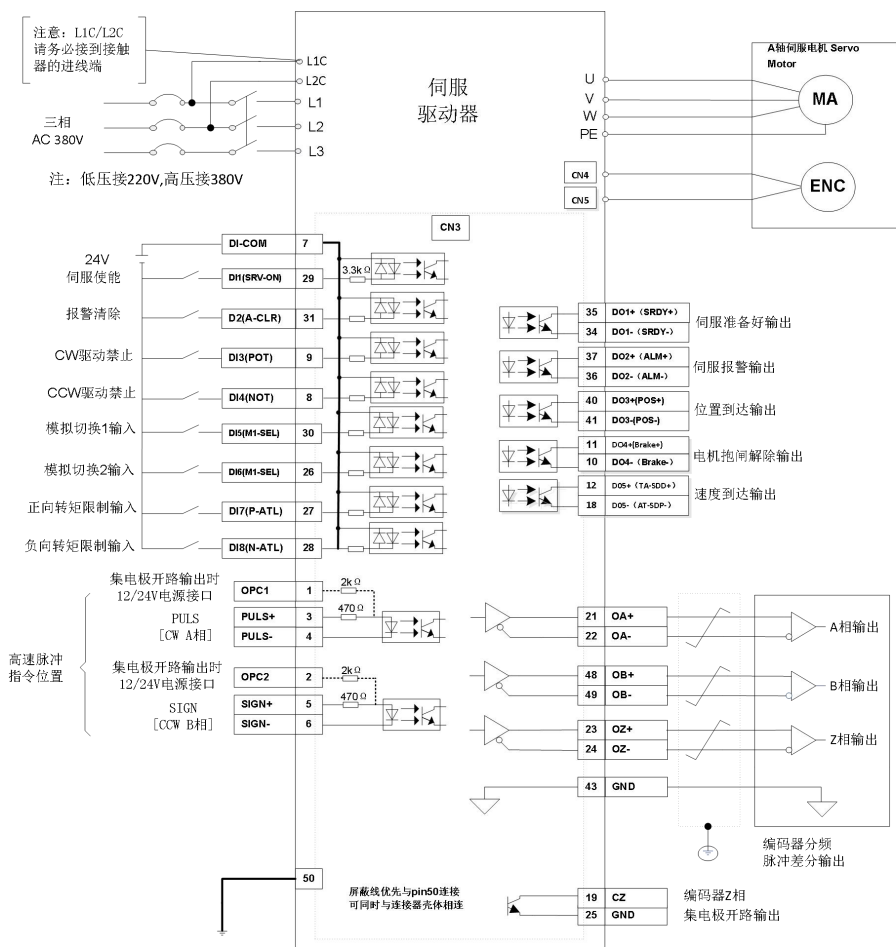
图 3-11 位置控制方式接线图
