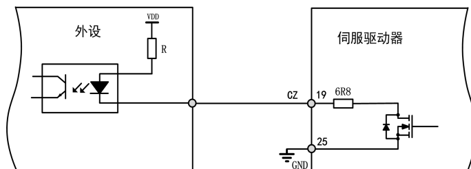
图 3-7 编码器 Z 信号集电极开路输出
