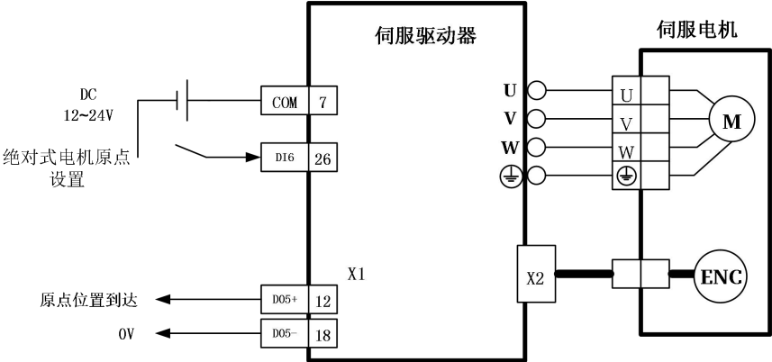
图 7-5 绝对式电机回零接线示意图
