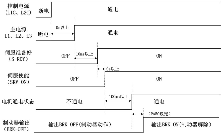
图 5-10 电源接通时接收伺服开启信号的时序
