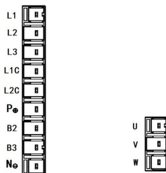
图 3-3 端子排分布图
